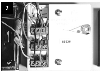
Anschluss Klingel max. 24V AC/DC. Anschluss Beleuchtung max. 12V AC/DC.
